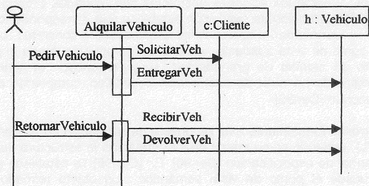
Figura no. 1 Sincronización abstracta para AlquilerVehiculo
